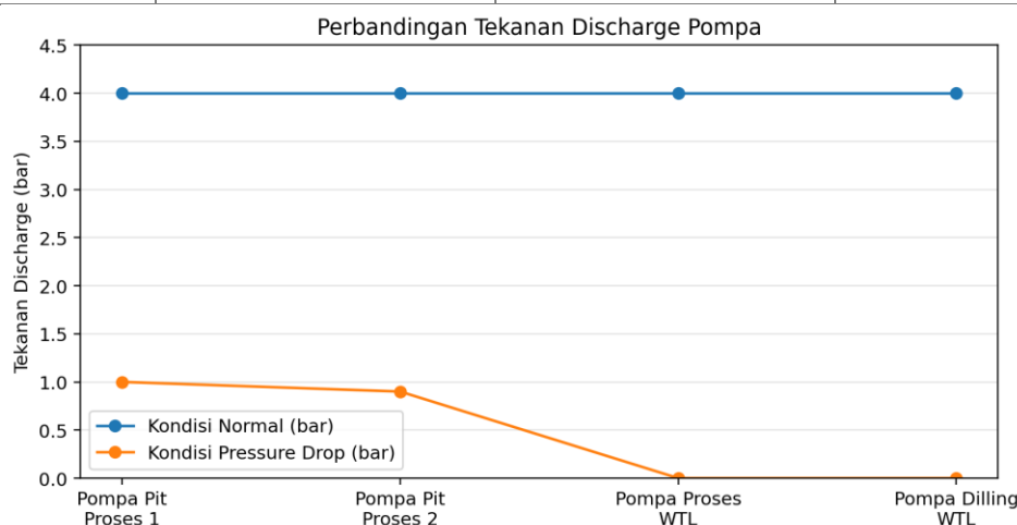
Gambar 5. Grafik perbandingan pressure discharge kondisi normal dan pressure drop
