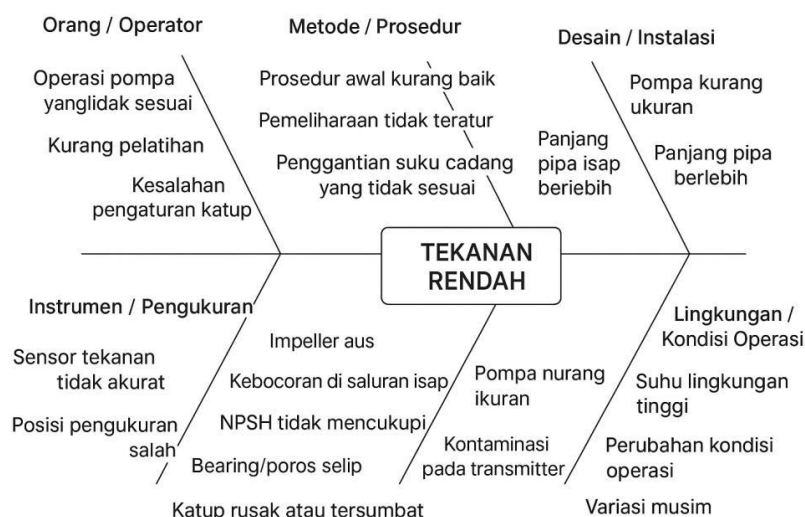
Gambar 2. Diagram fishbone analisis penyebab pressure drop pada sistem pompa sentrifugal
