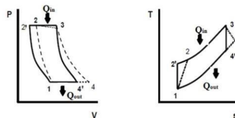
Gambar 5. Urutan Siklus Brayton
