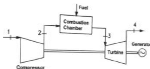
Gambar 6. Skema Siklus Turbin Gas
