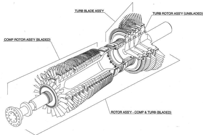
Gambar 3. Komponen Pada Gas Turbin
