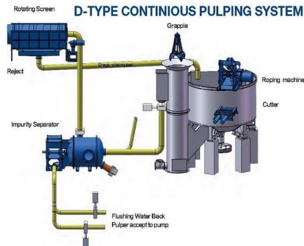
Gambar 2. Skematik Mesin Drum Pulper
