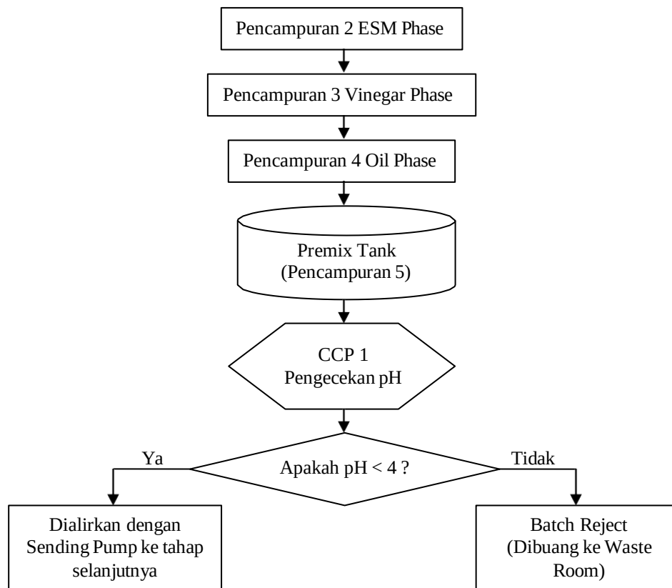
Gambar 2. Diagram Alir CCP 1 (Pencampuran 5)
