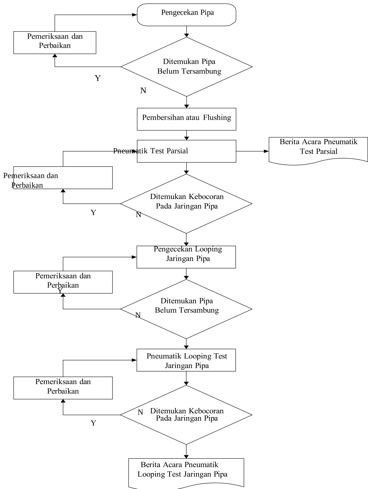
Gambar 2. Flowchart proses pengujian pneumatic pada pipa PE distribusi 180 mm.
