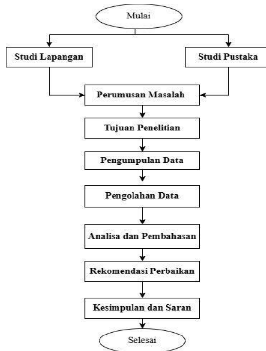
Gambar 1. Tahapan penelitian
