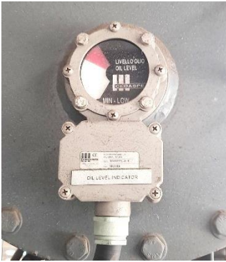
Gambar 9. Oil Level Indicator yang berada di samping tangki konservator
