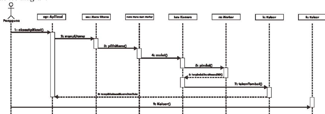
Gambar 3. Sequence Diagram Aplikasi
